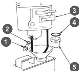
Рис. 28 Обслуживание фильтра-отстойника
