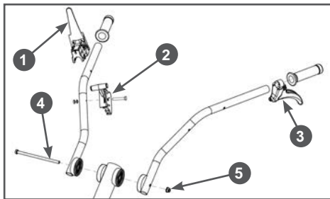
Рис. 7 Установка рукояток управления
