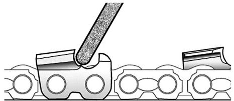
Рис. 16 Регулировка глубины заточки
