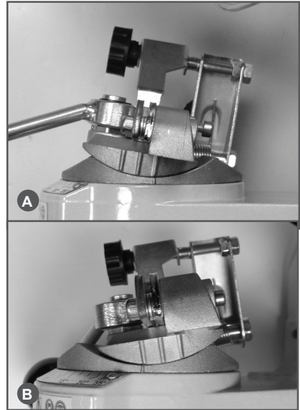
Рис. 15 Установка угла поперечного наклона
