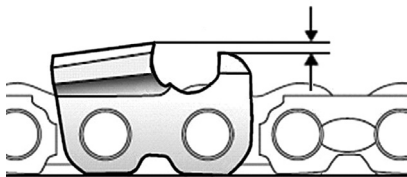
Рис. 22 Глубина резания
