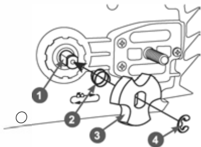
Рис. 23 Снятие ведущей звездочки 1. Вал шестерни 2. Пружина 3. Звездочка 4. Кольцо стопорное
