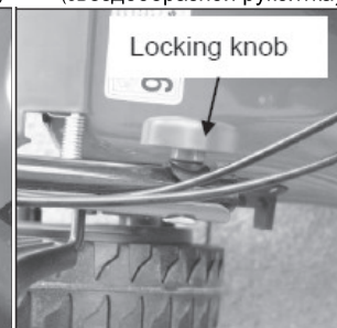
Рис.2С (Контргайка)
