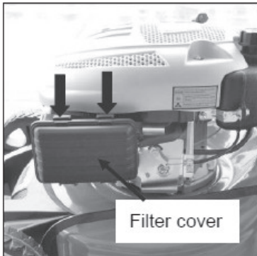
Рис.15А (Крышка фильтра)
