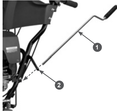
Рис. 26 Установка рычага управления поворотом жёлоба
